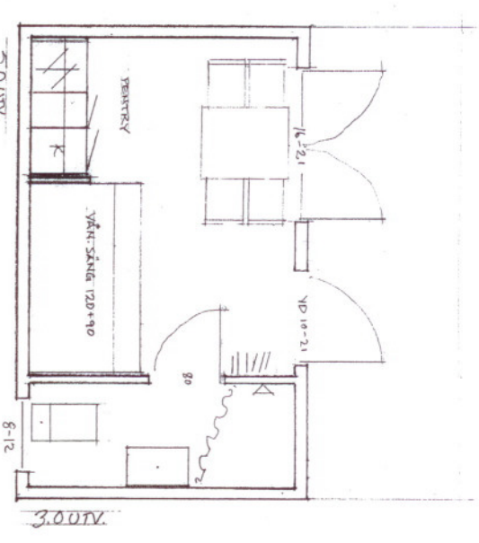
PLAN ISH UTV. 1:50
